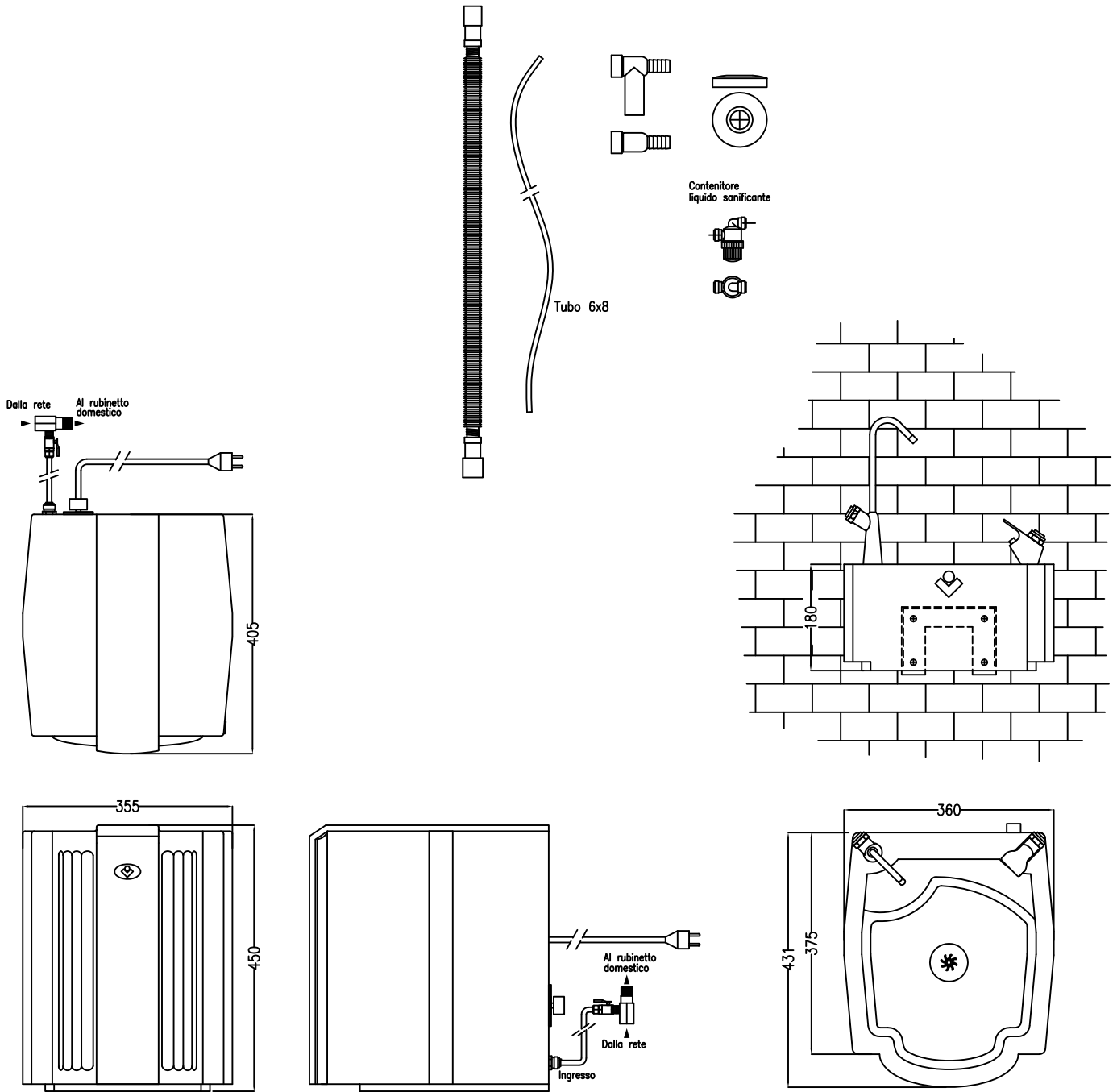
FONTESANA GRUPPO REFRIGERATORE SPRINGER-Cod.12813AA
